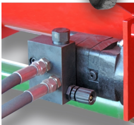
ACIONAMENTO HIDRÁULICO
